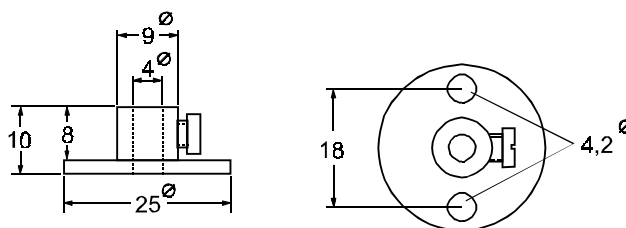
Montageflansch MF4
